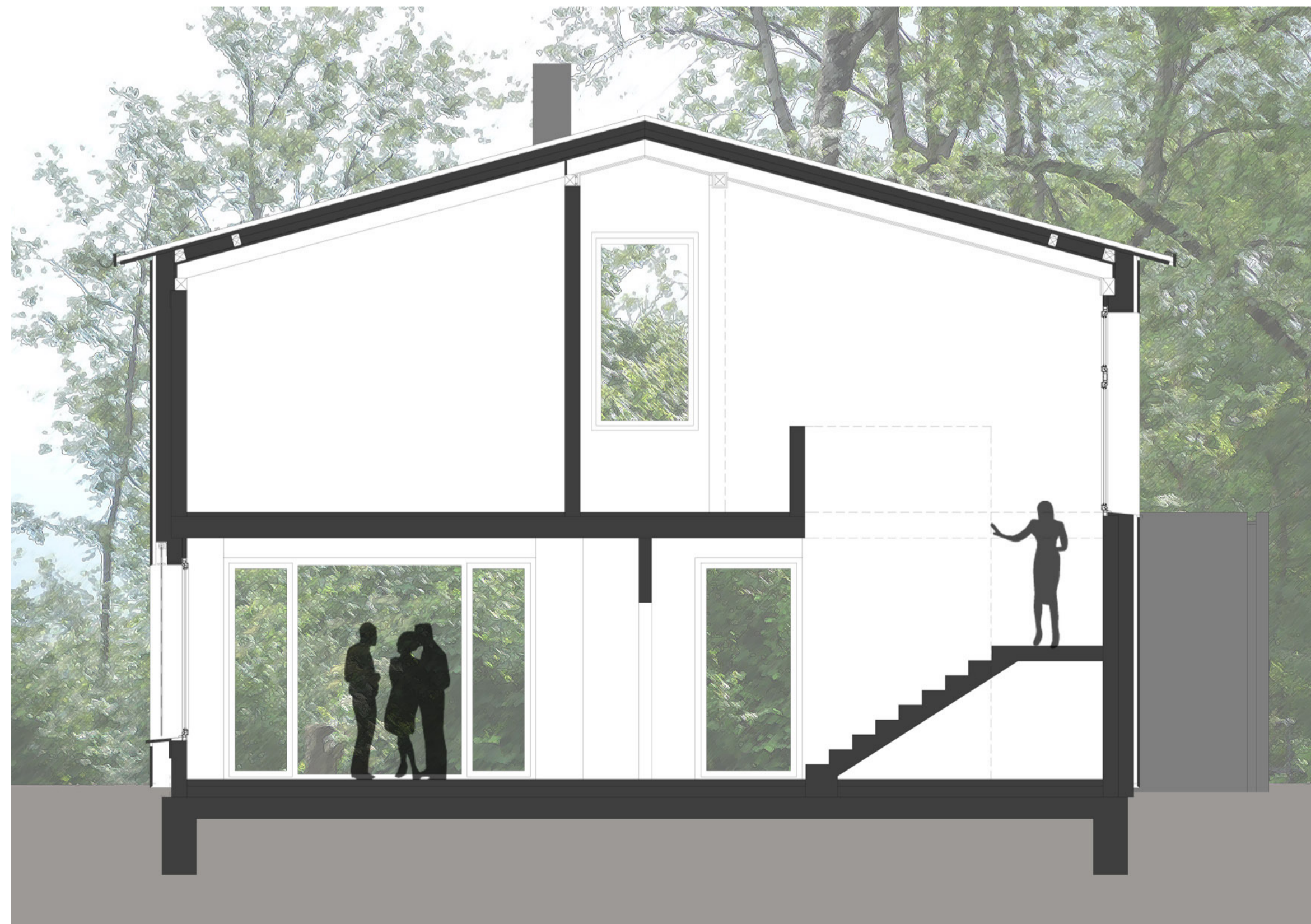
Querschnitt
