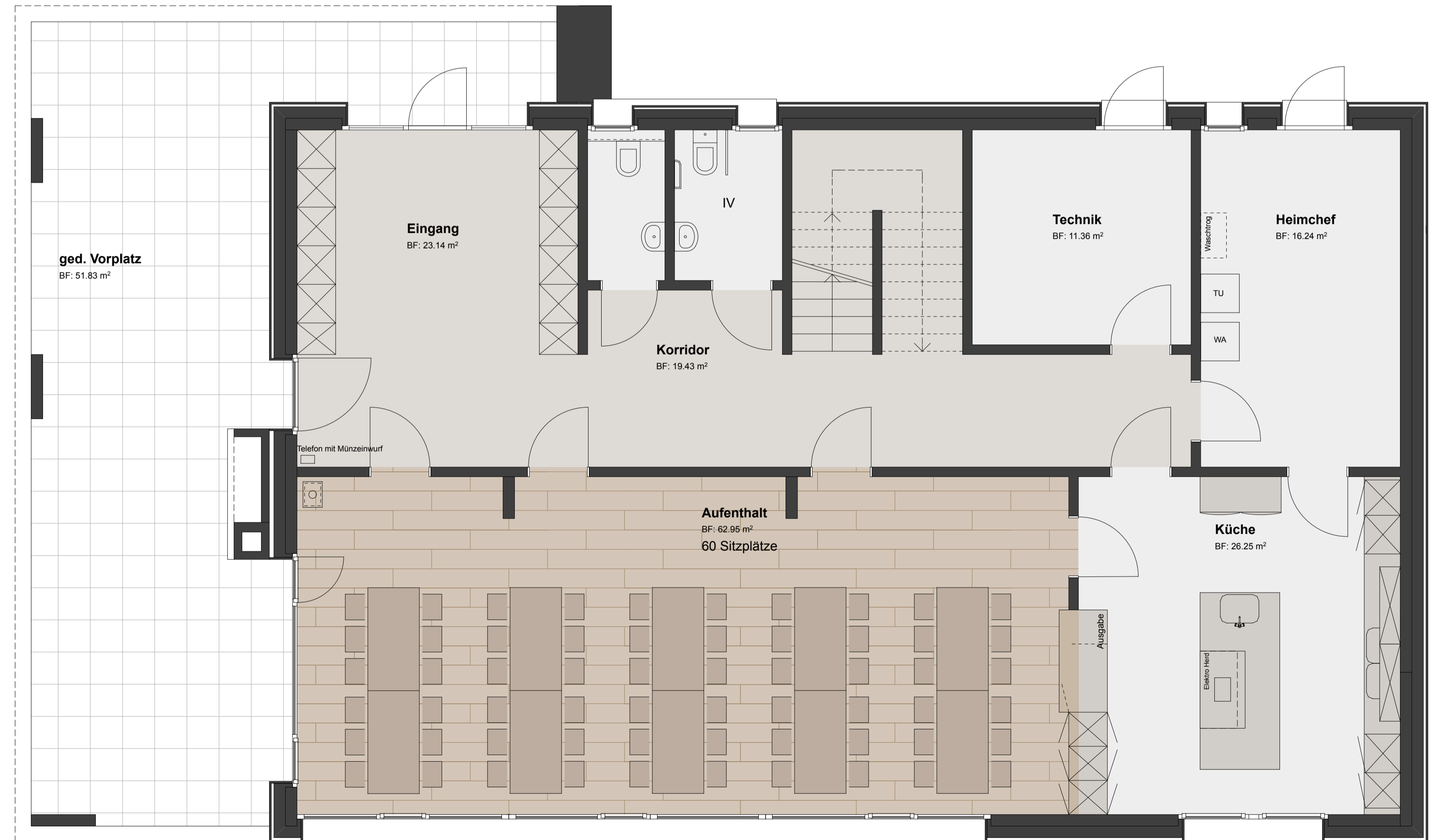
Erdgeschoss
